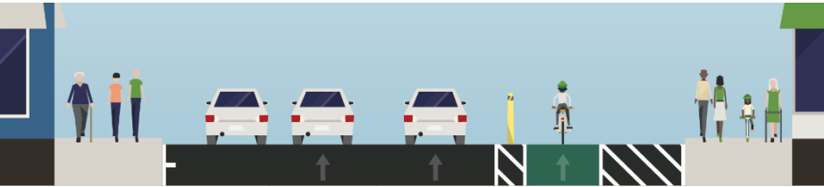
GOLDEN GATE建議街道剖面圖
