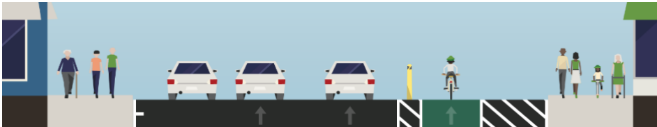
MGA MUNGKAHING CROSS-SECTION (MGA ELEMENTONG TULAD NG MGA LANE, SHOULDER, AT SLIDESLOPE) SA GOLDEN GATE AVENUE
