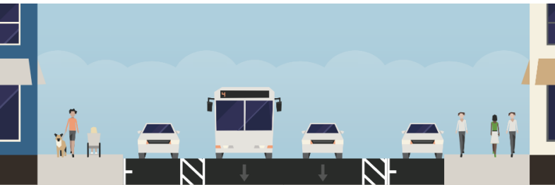
MGA MUNGKAHING CROSS-SECTION (MGA ELEMENTONG TULAD NG MGA LANE, SHOULDER, AT SLIDESLOPE) SA LEAVENWORTH
